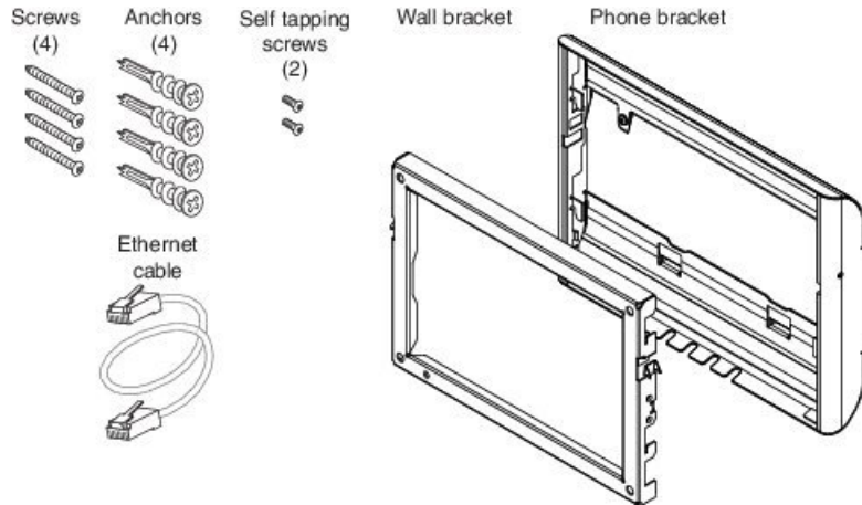
Şekil 20: 7861 için Duvar Montaj Kiti Bileşenleri
