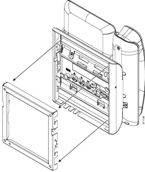
Şekil 17: Telefonun Duvar Desteğine Takılması
