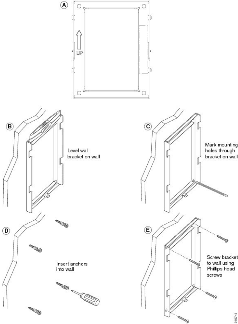
Şekil 5: Destek Kurulumu
