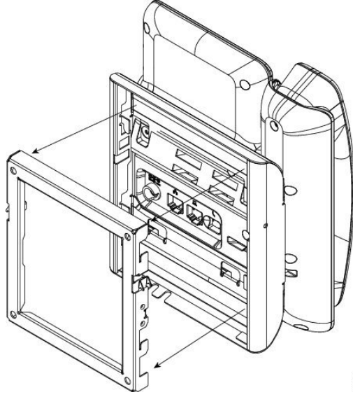
Şekil 8: Telefonun Duvar Desteğine Takılması
