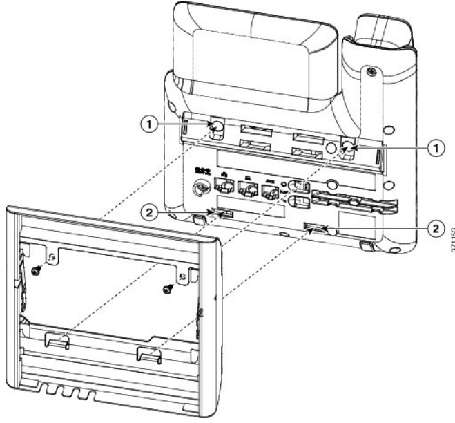
Şekil 15: Telefon Desteğinin Takılması
