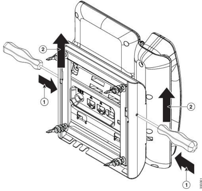
Şekil 10: Tırnakları Serbest Bırakma
