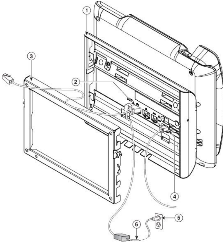
Şekil 25: Kablonun Takılması
