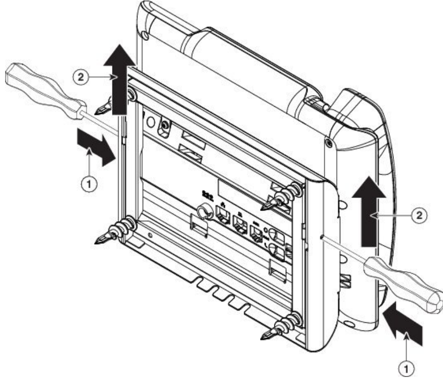
Şekil 28: Tırnakları Serbest Bırakma
