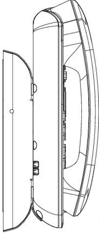
Şekil 22: Telefona Kurulan ADA Kilitlenmeyen Duvar Montaj Kitinin Yandan Görünümü
