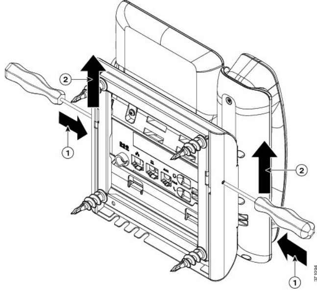
Şekil 19: Tırnakları Serbest Bırakma
