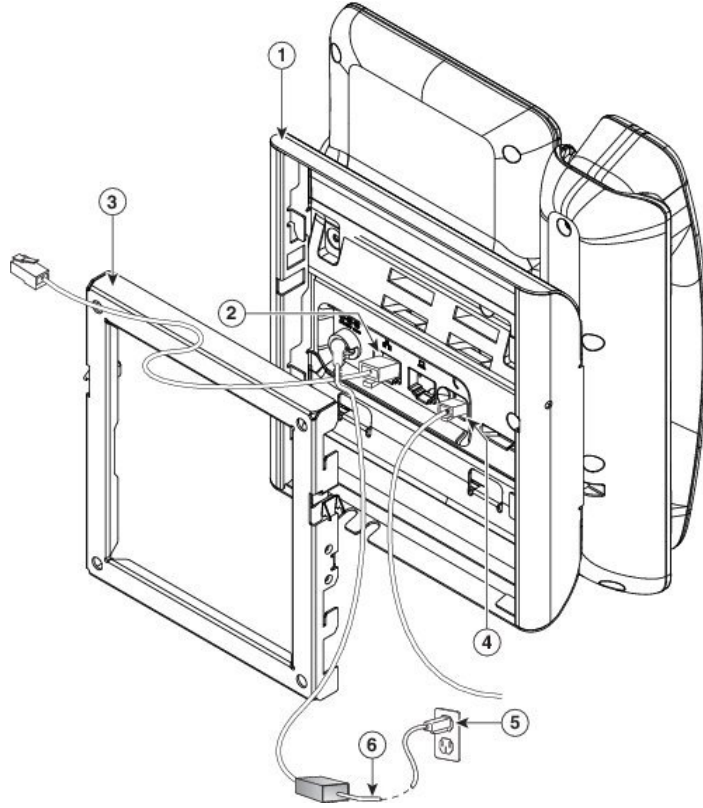
Şekil 7: Kablonun Takılması
