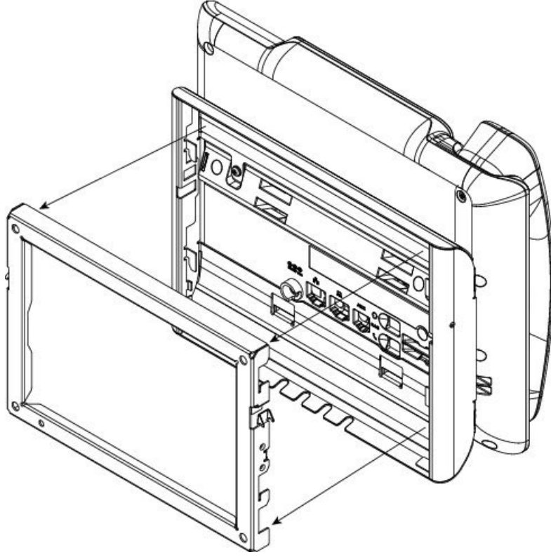
Şekil 26: Telefonun Duvar Desteğine Takılması
