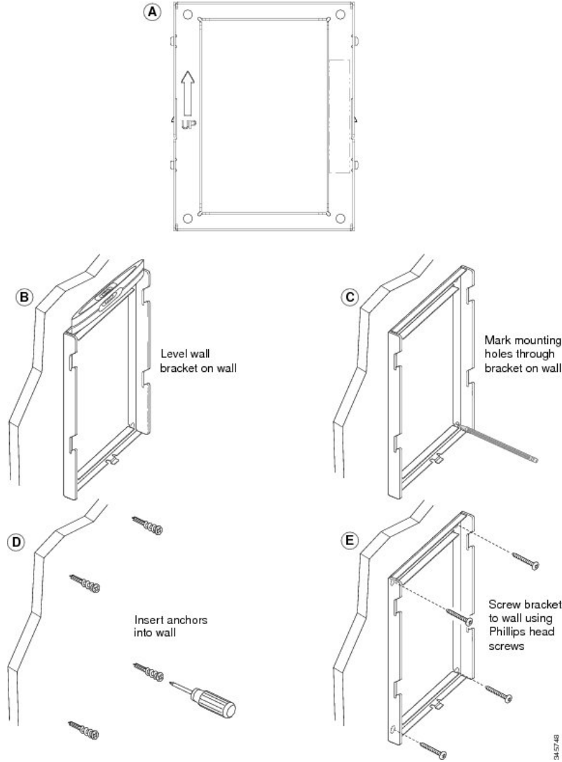
Şekil 14: Destek Kurulumu
