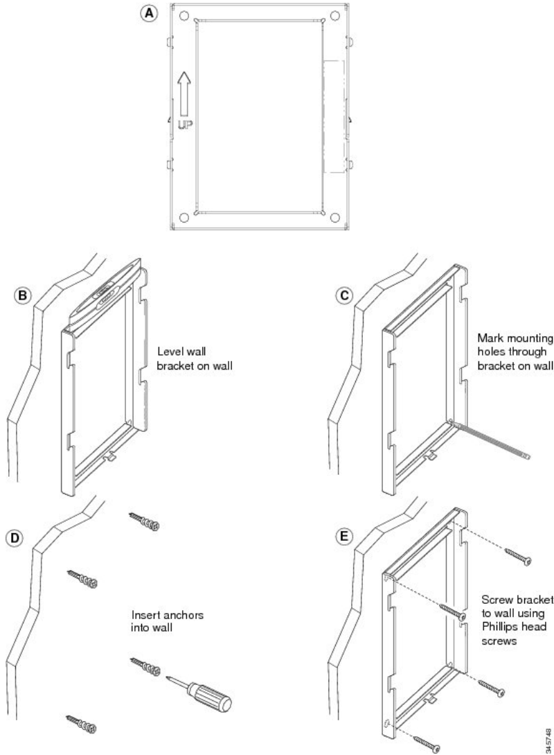
Şekil 23: Destek Kurulumu
