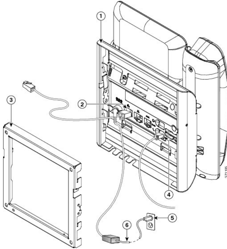
Şekil 16: Kablonun Takılması
