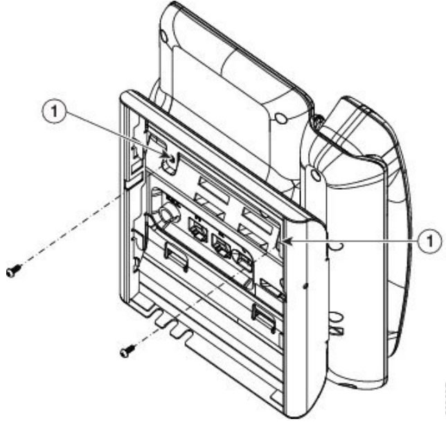
Şekil 6: Telefon Desteğinin Takılması
