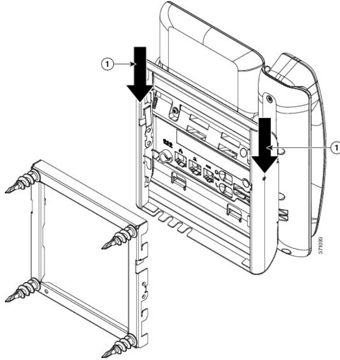
Şekil 18: Tırnağın Konumu
