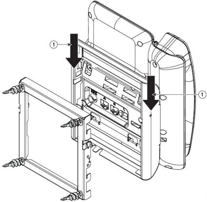
Şekil 9: Tırnağın Konumu
