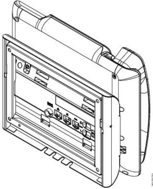
Şekil 21: Telefona Kurulan ADA Kilitlenmeyen Duvar Montaj Kitinin Arkadan Görünümü
