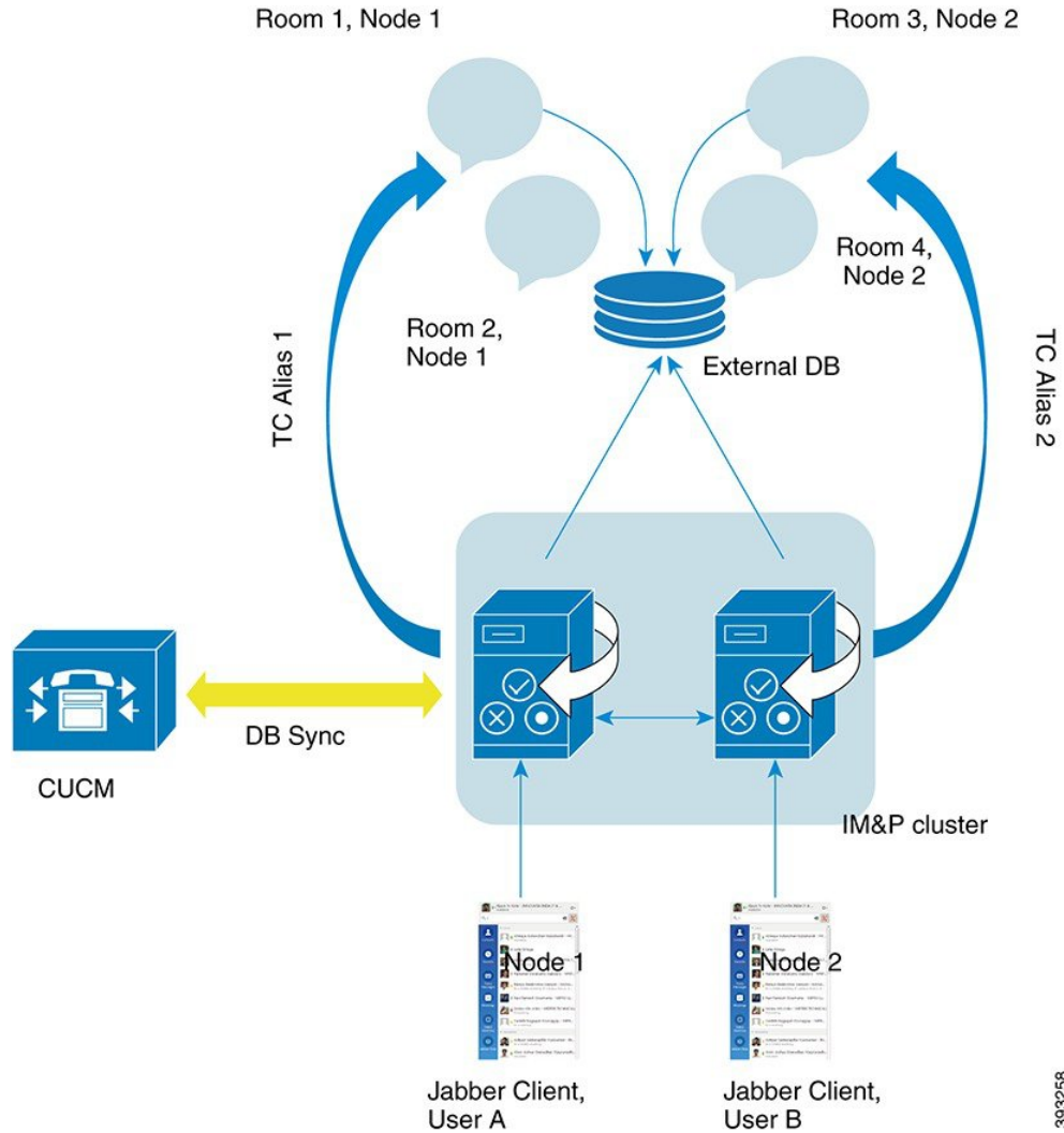
图 6: 永久聊天高可用性结构
