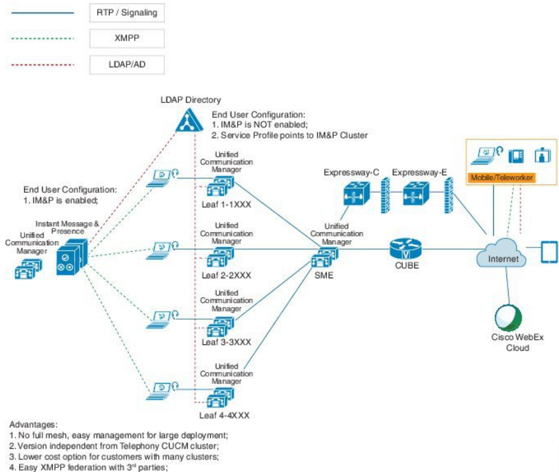
图 3: IM and Presence 服务集中式群集架构
