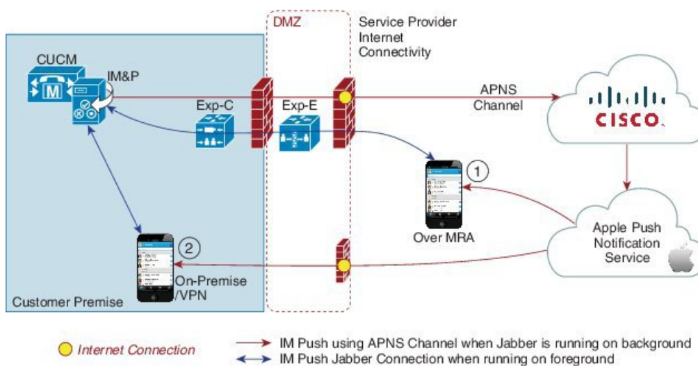
图 5: iPhone 和 iPad 版 Cisco Jabber 的推送通知架构
