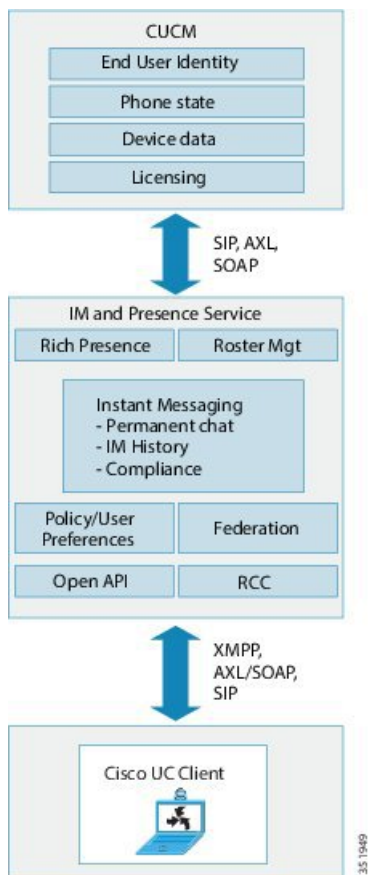
图 1: IM and Presence 服务基本部署
