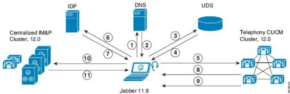
图 4 IM and Presence 服务集中式群集使用案例
