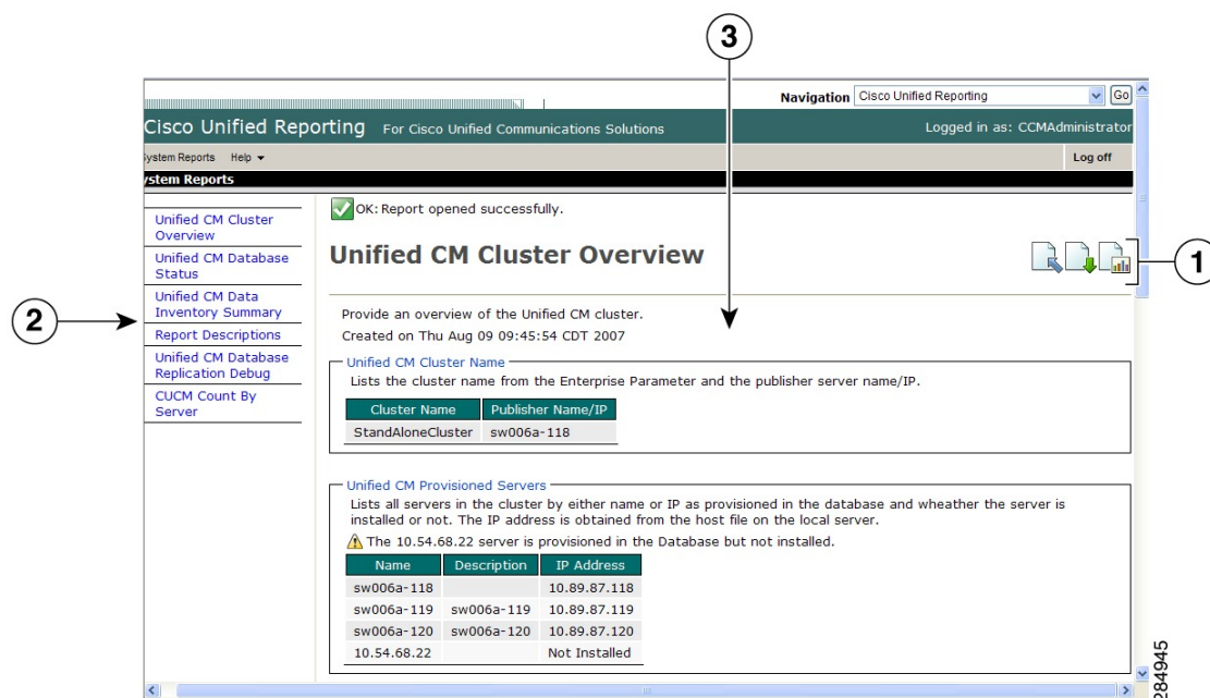
圖 23: UI 元件
