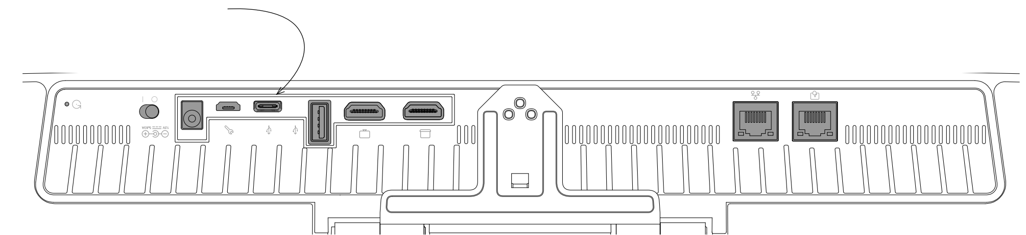
將電腦連接至 USB-C 插槽
