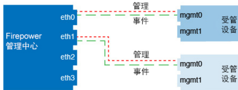
图 19: Firepower 管理中心上的多个管理接口
