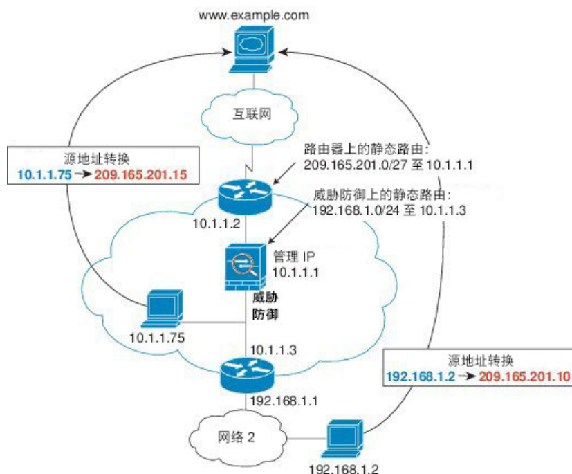
图 23: NAT 示例：透明模式
