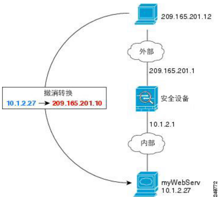
图 35: 面向内部 Web 服务器的静态 NAT
