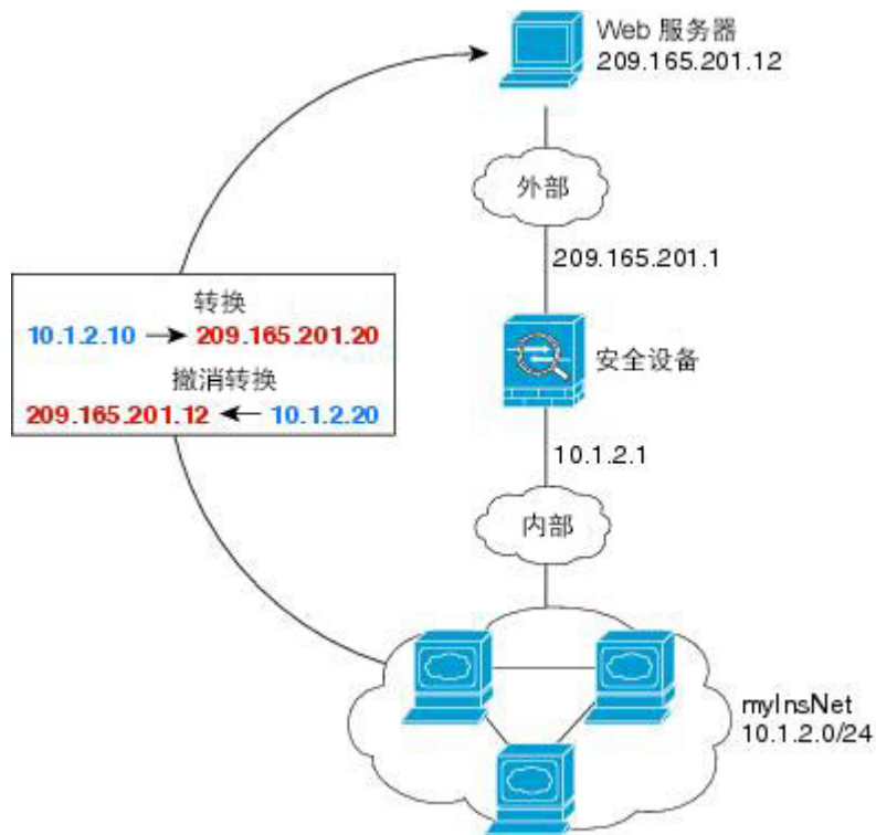
图 36: 面向内部 Web 服务器的动态 NAT, 面向外部 Web 服务器的静态 NAT
