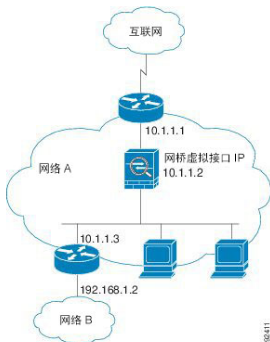
图 2: 透明防火墙网络
