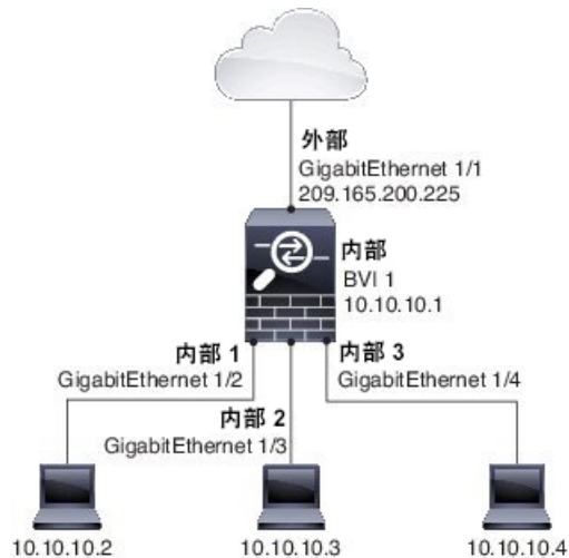
图 4: 具有内部网桥组和外部路由接口的路由防火墙网络
