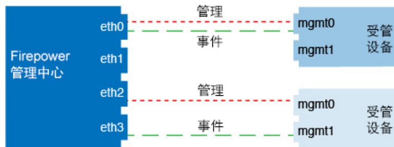
图 21: 混合管理和事件接口用法
