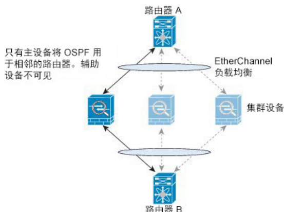
图 15: 动态路由
