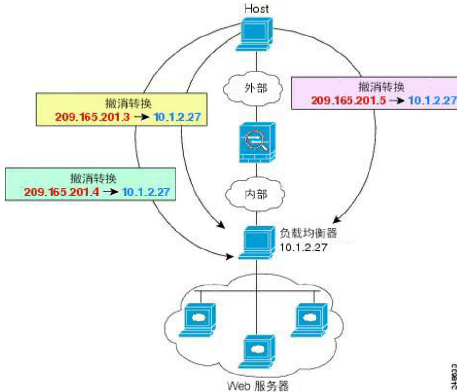
图 37: 内部负载均衡器的一对多静态 NAT
