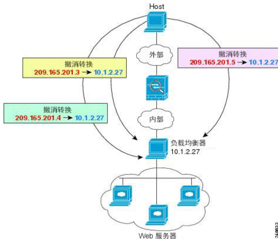
图 31: 一对多静态 NAT 示例
