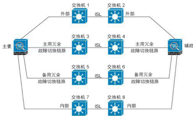
图 14: 使用交换机间链路连接
