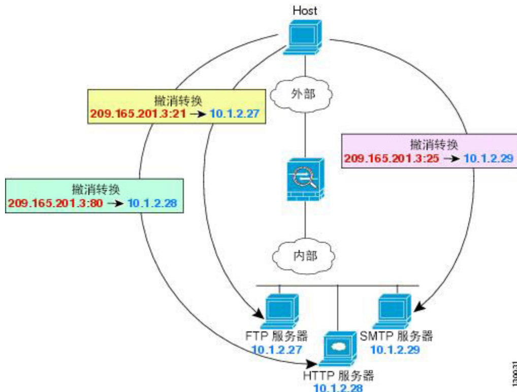
图 38: 支持端口转换的静态 NAT
