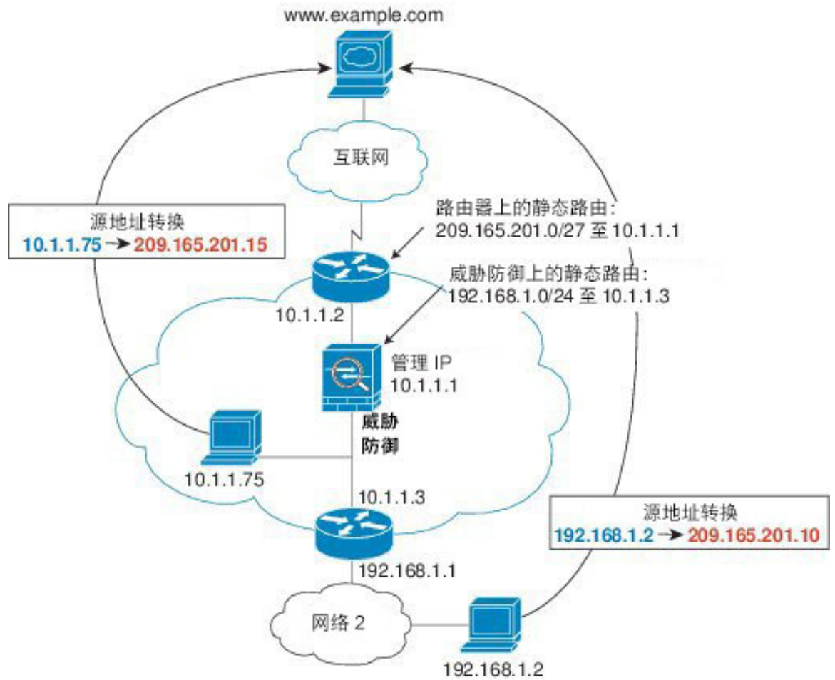
图 5: NAT 示例：网桥组中的 NAT
