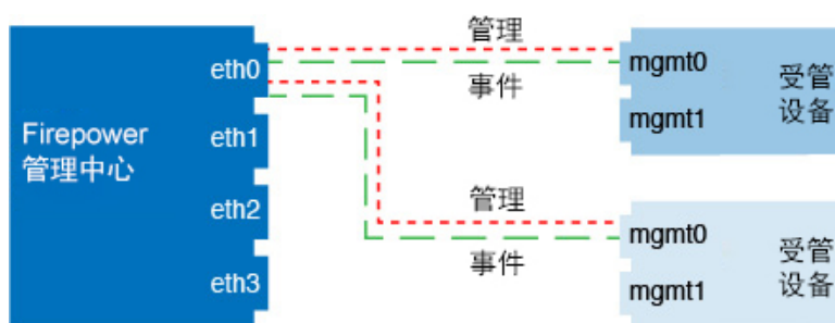
图 18: Firepower 管理中心上的单个管理接口
