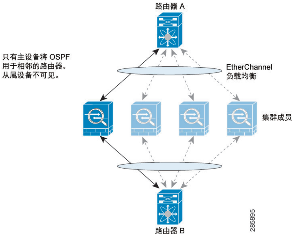
图 17: 集群下的动态路由
