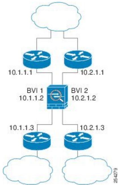
图 3: 具有两个网桥组的透明防火墙网络
