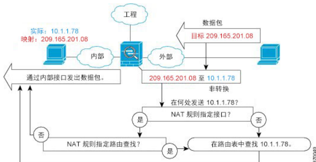
图 16: 含 NAT 的路由模式出口接口选择
