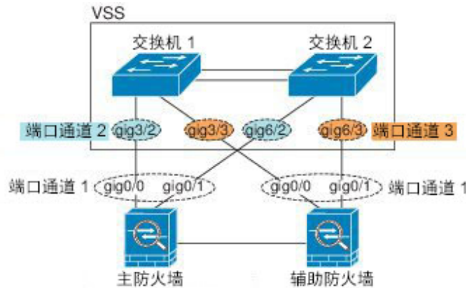
图 7: 主用/备用故障切换和 VSS/vPC
