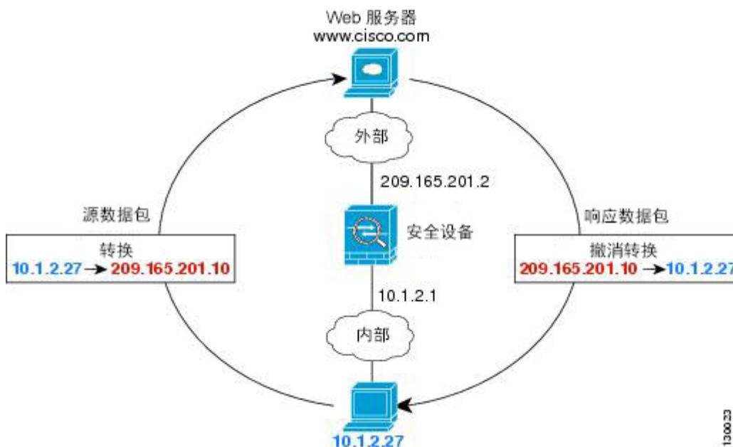
图 22: NAT 示例：路由模式
