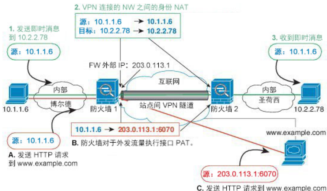
图 41: 用于站点到站点 VPN 的接口 PAT 和身份 NAT
