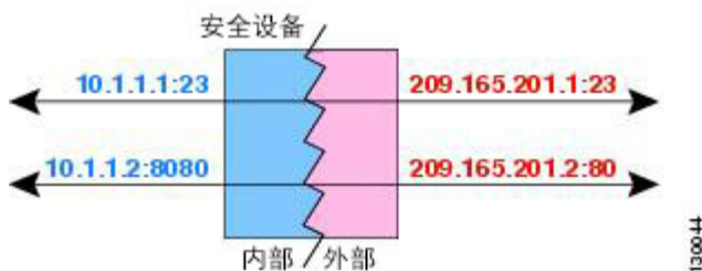
图 29: 支持端口转换的典型静态 NAT 场景
