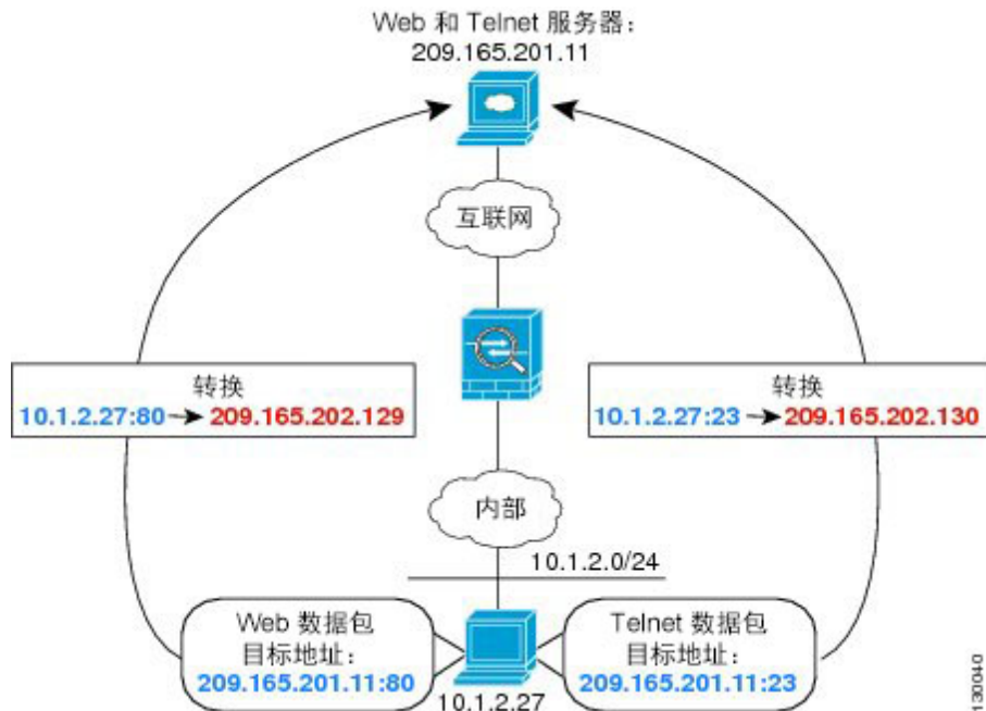
图 40: 具有不同目标端口的手动 NAT
