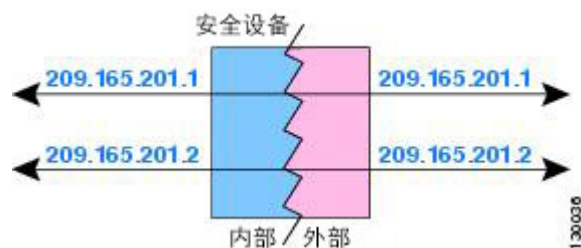
图 34: 身份 NAT
