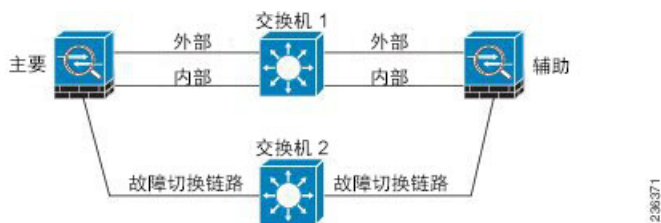
图 11: 通过电缆连接
