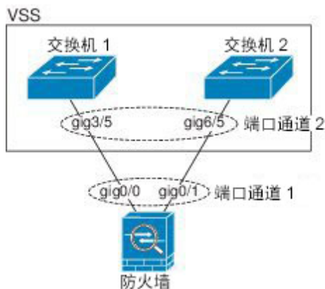
图 6: 连接至 VSS/vPC
