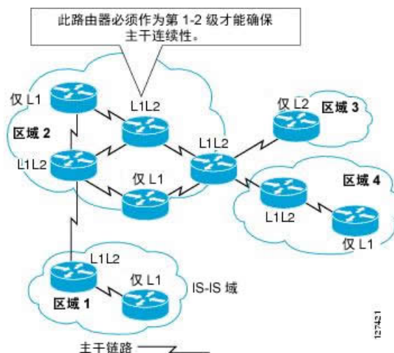
图 71: IS-IS 网络拓扑中的级别 1、级别 2、级别 1-2 设备
