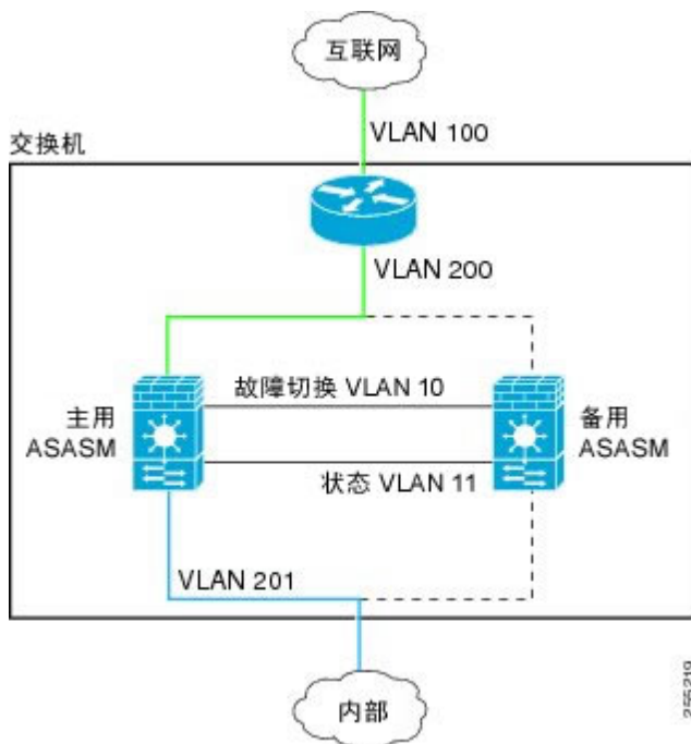
图 52: 交换机内故障切换
