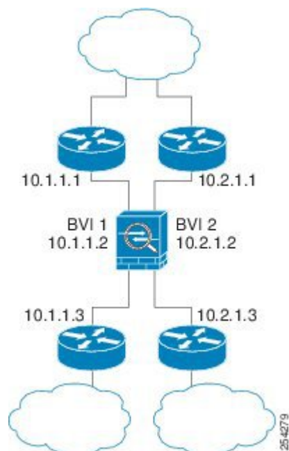
图 25: 具有两个网桥组的透明防火墙网络
