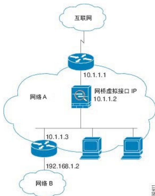
图 24: 透明防火墙网络
