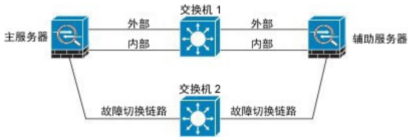
图 48: 通过电缆连接
