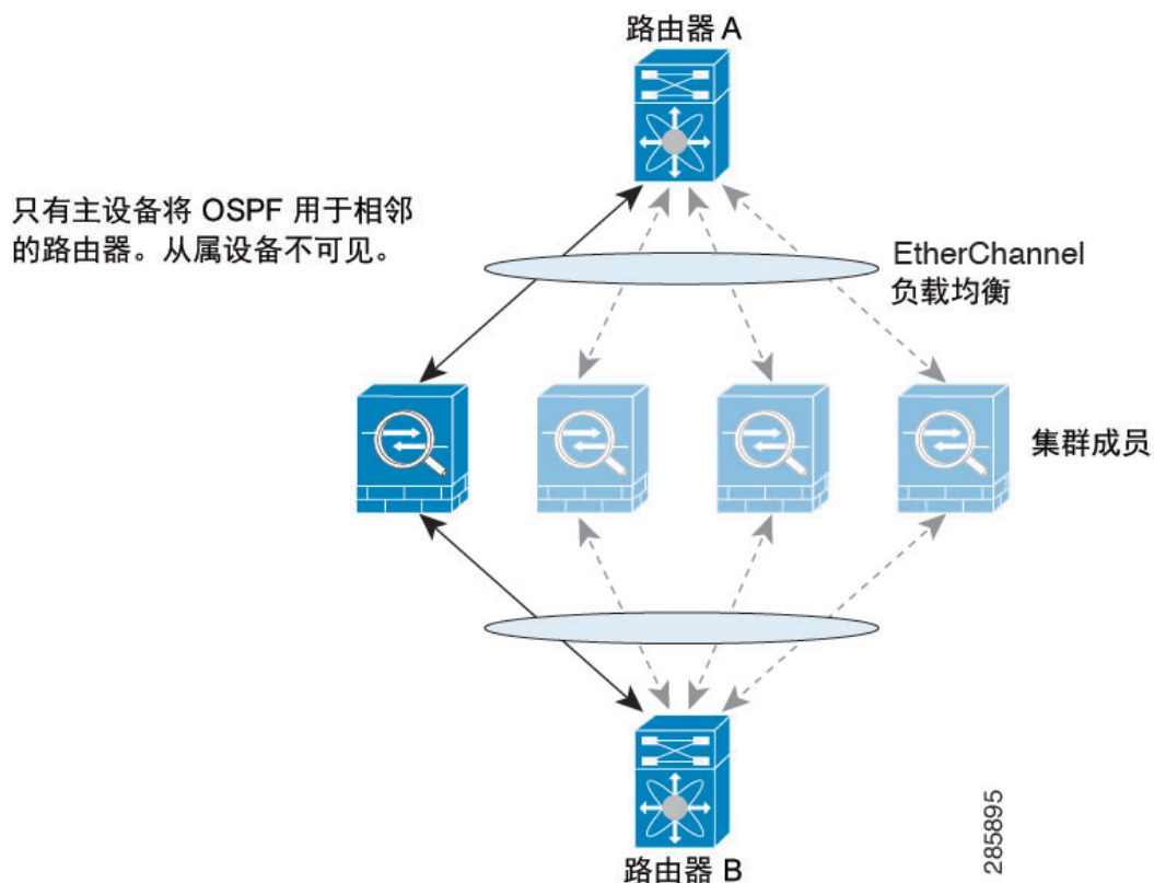
图 66: 跨网络 EtherChannel 模式下的动态路由
