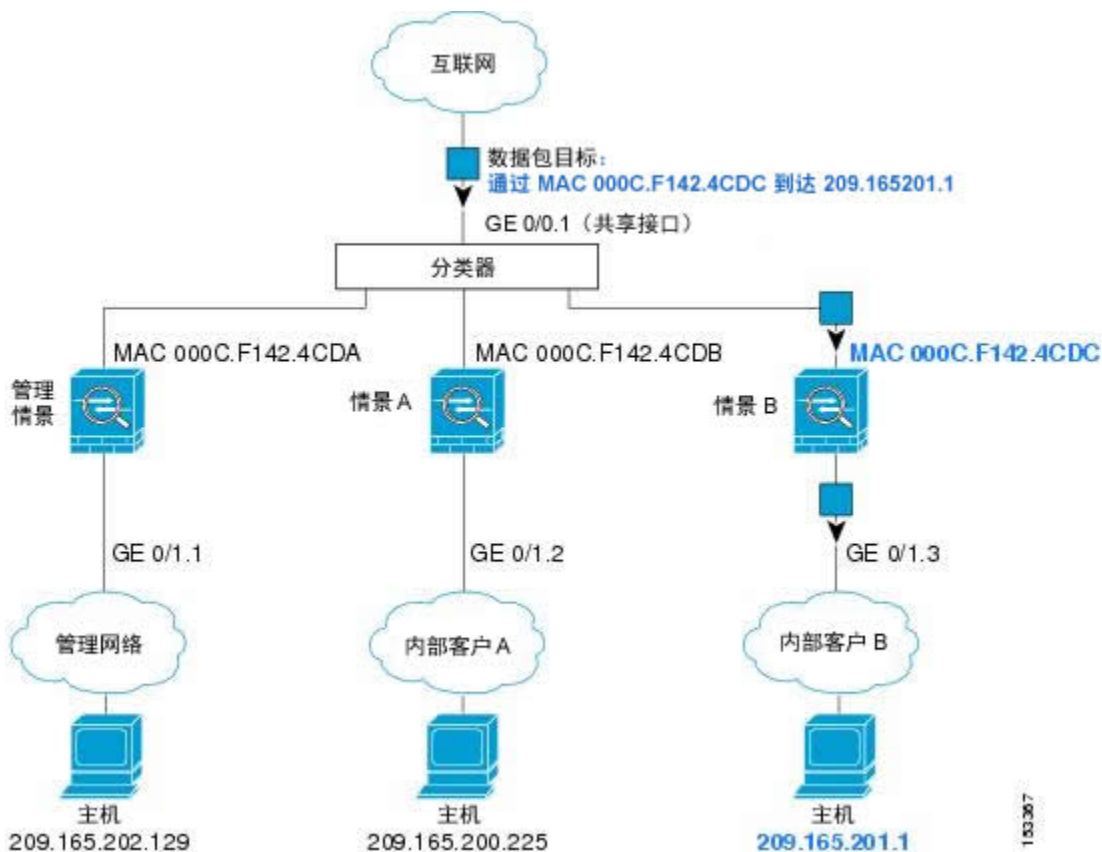
图 38: 使用 MAC 地址通过共享接口进行数据包分类
