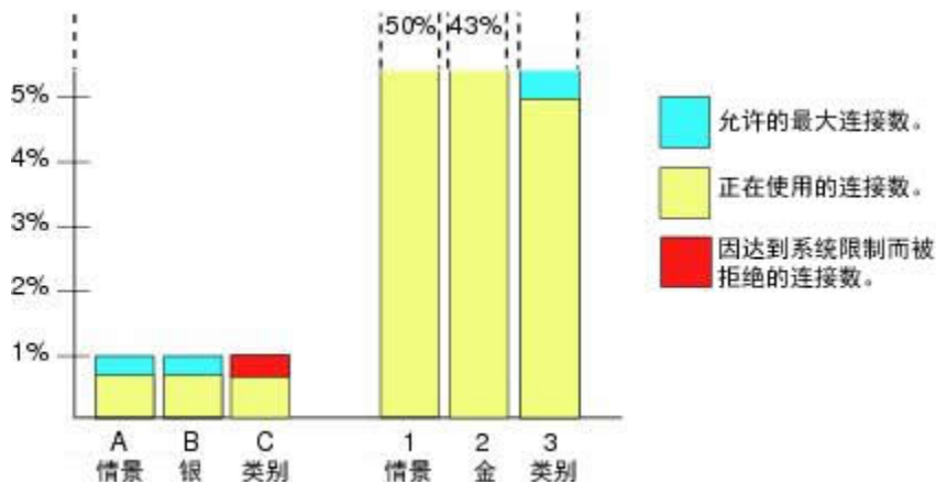
图 44: 不受限制的资源
