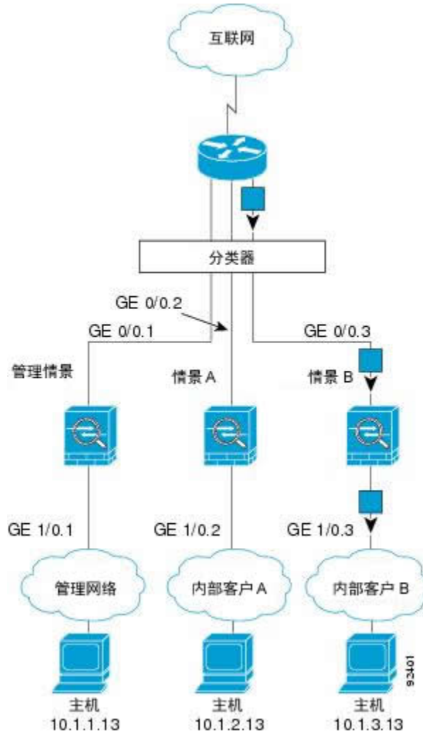
图 40: 透明防火墙情景
