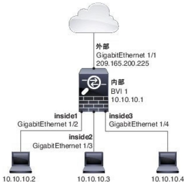
图 26: 具有内部网桥组和外部路由接口的路由防火墙网络
