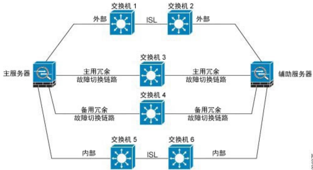
图 51: 使用交换机间链路连接
