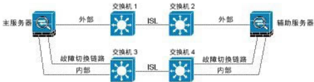
图 49: 使用安全交换机连接
