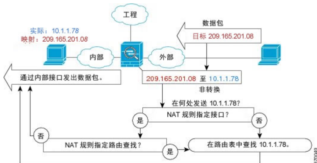
图 65: 含 NAT 的路由模式出口接口选择
