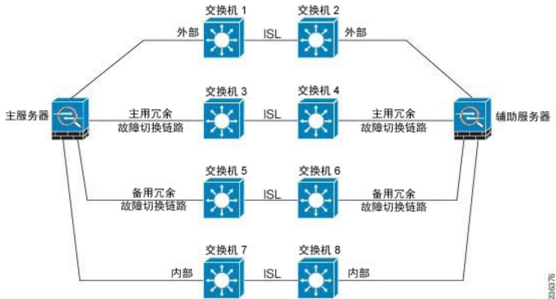
图 51: 使用交换机间链路连接
