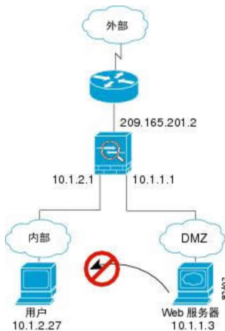
图 32: 从 DMZ 到内部
