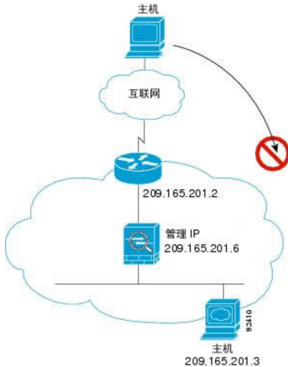
图 37: 从外部到内部
