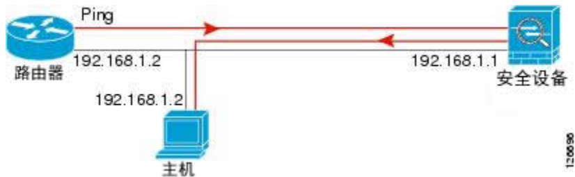
图 81: IP 寻址问题引发的 ping 故障
