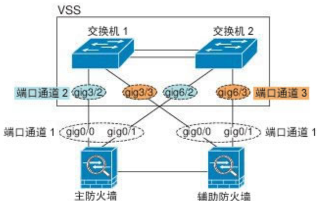
图 63: 主用/备用故障切换和 VSS/vPC
