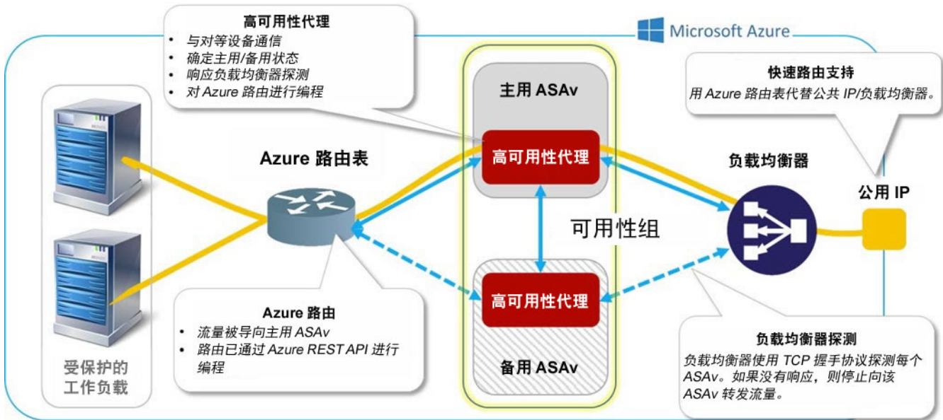
图 58: Azure 中的 ASA 高可用性部署
