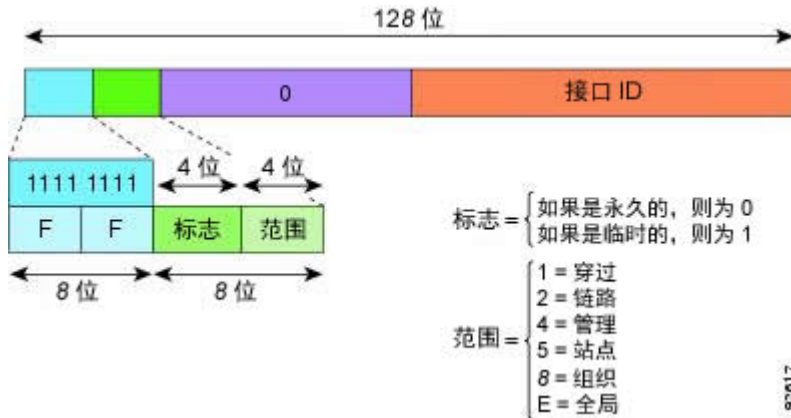
图 84: IPv6 组播地址格式
