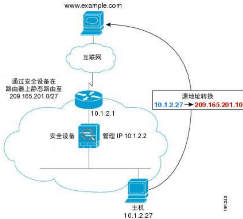
图 35: 使用 NAT 从内部到外部
