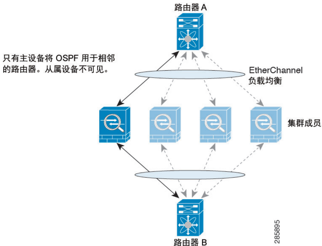
图 59: 跨网络 EtherChannel 模式下的动态路由
