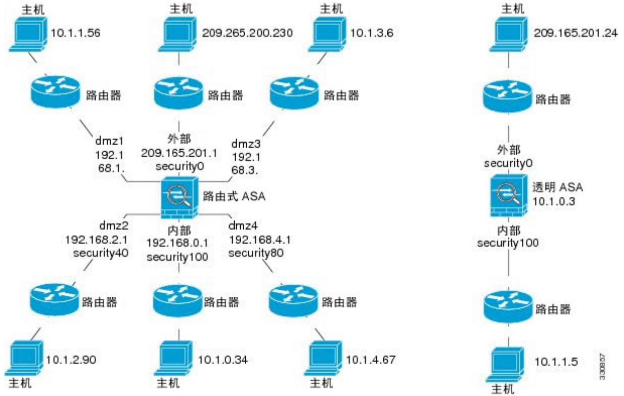
图 79: 接口、路由器和主机的网络图
