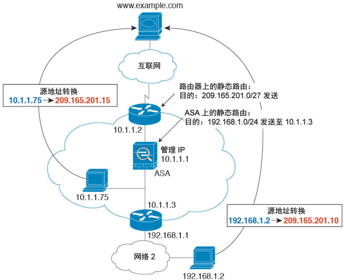
图 27: NAT 示例：网桥组中的 NAT
