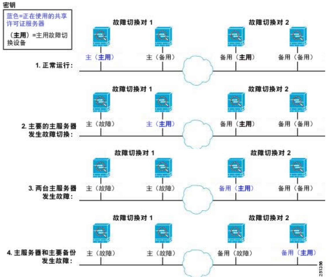
图 13: 故障切换和共享许可证服务器
