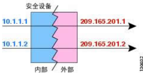
图 18: 动态 NAT
