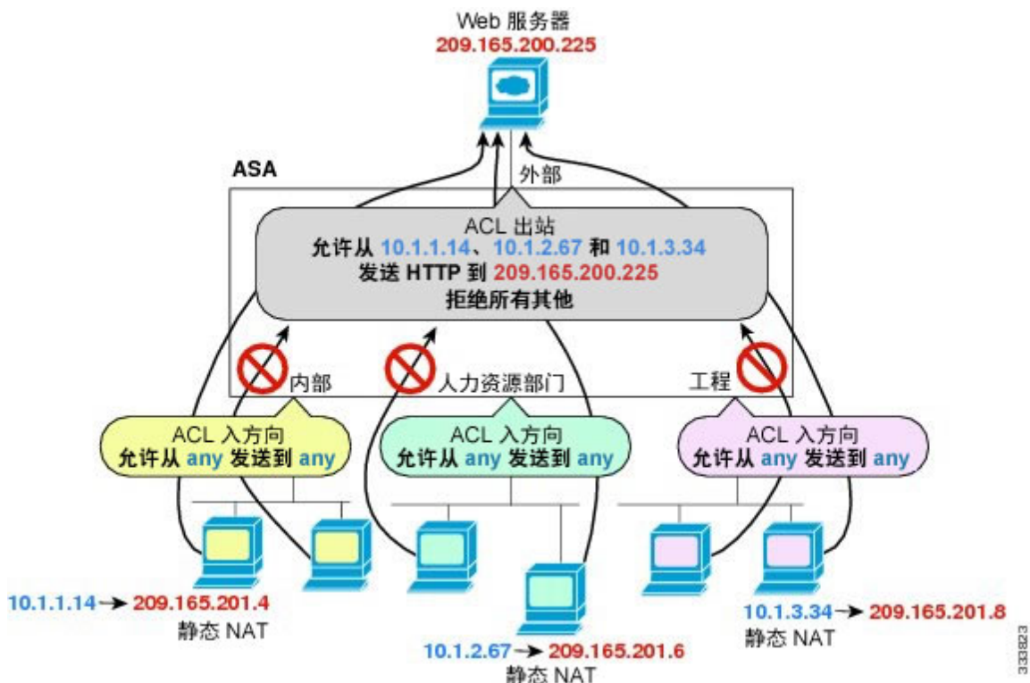
图 2: 出站 ACL
