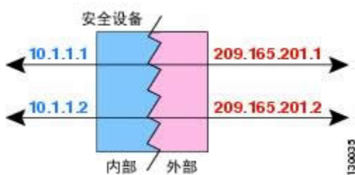
图 21: 静态 NAT
