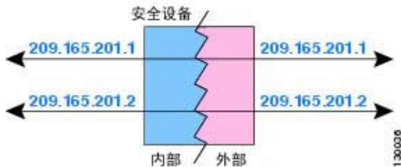
图 27: 身份 NAT
