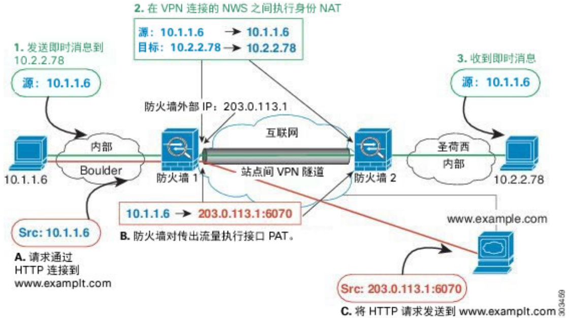
图 42: 用于站点到站点 VPN 的接口 PAT 和身份 NAT
