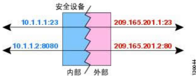
图 22: 支持端口转换的典型静态 NAT 场景
