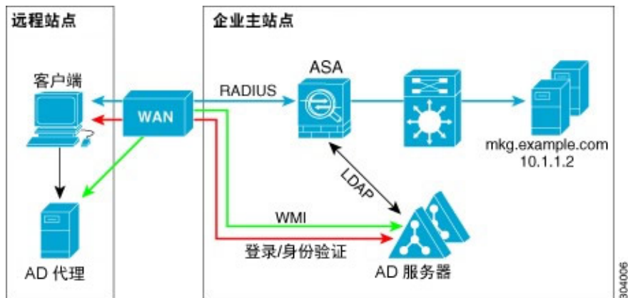
图 8: 具有远程 AD 代理的基于广域网的部署
