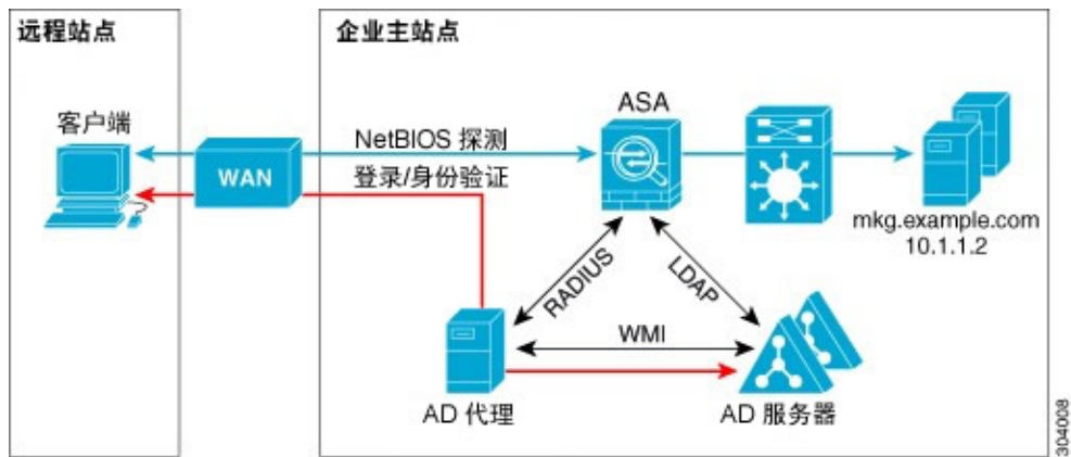
图 7: 基于广域网的部署
