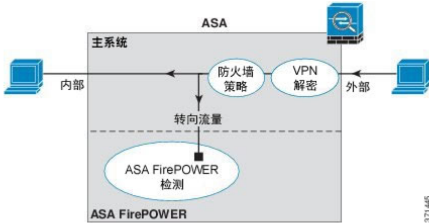
图 14: ASA FirePOWER 内联分路仪监控模式
